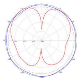
1710-2700MHz
